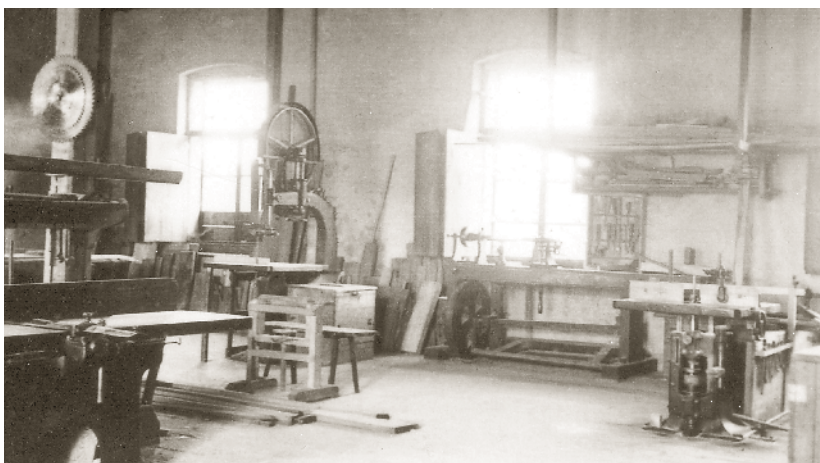
Mizarska delavnica Karla Jevščka je bila ena redkih, ki je bila že pred 1. svetovno vojno opremljena s stroji. Pred 2. svetovno vojno je bila prenovljena, opremili so jo tudi z več novimi stroji. Na desni je mizni rezkar, ob oknu stružnica in orodje, ki ga je uporabljal strugar, levo ob oknu tračna žaga, skrajno levo pa poravnalnik. Nad njim visi rezilo za vzdolžno žaganje (foto: arhiv družine Jevšček).
